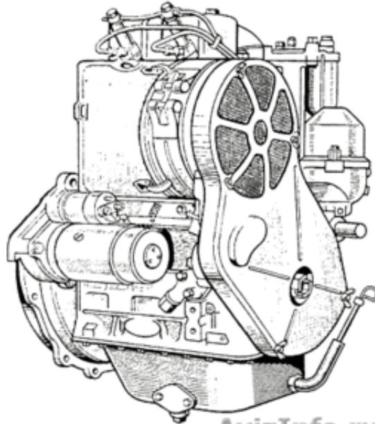
Рис. 2. Двигатель Д21 (вид справа)
